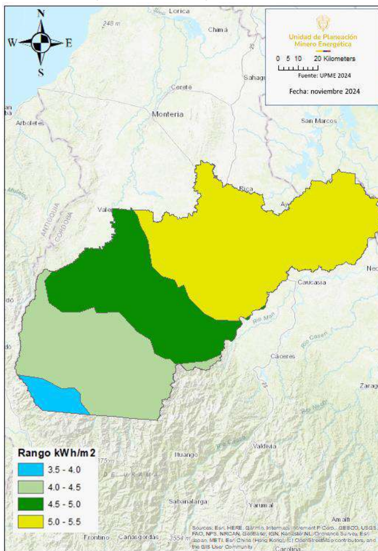
Ilustración 110. Potencial generación de energía solar en el distrito del Sur de Córdoba.
