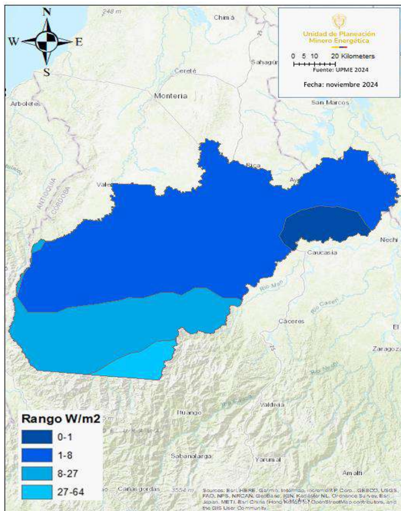
Ilustración 113. Potencial generación de energía eólica a 20 m de altura en el Sur de Córdoba.
