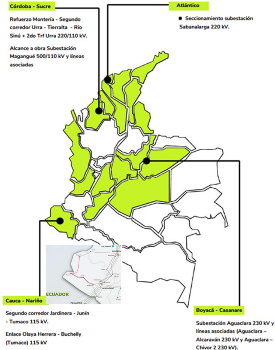
Ilustración 92. “Segundo corredor Jardinerá-Junín-Buchelly (Tumaco) 115 kV” en el segundo paquete de obras urgentes 2024.
