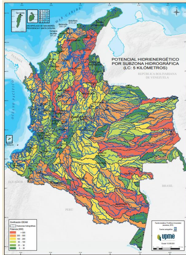
Ilustración 86. Potencial hidroenergético en Colombia por subzona hidrográfica Lc:5km.
