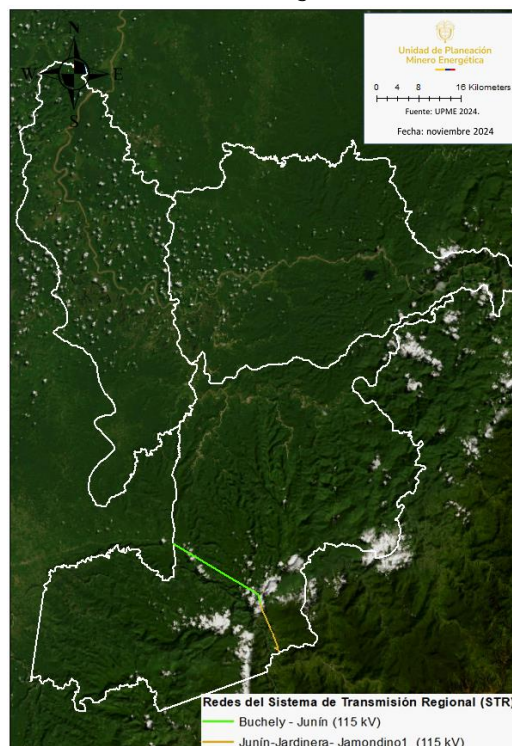
Ilustración 91. Redes de Sistema de Transmisión Regional (STR) en el distrito del Triángulo de Telembí.
