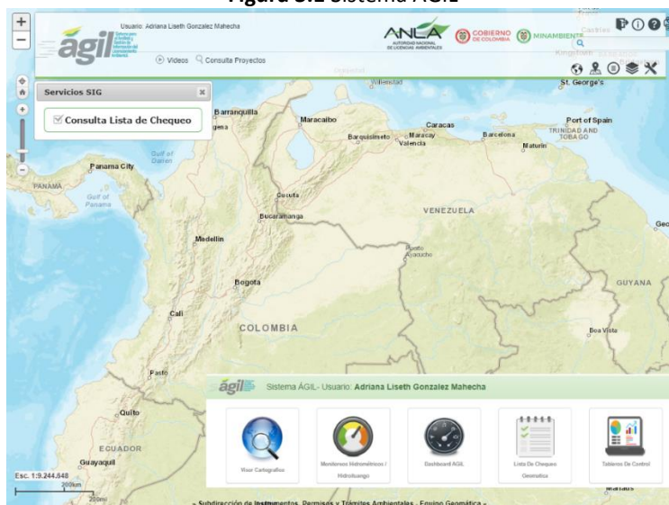
Figura 3.1 Sistema ÁGIL
