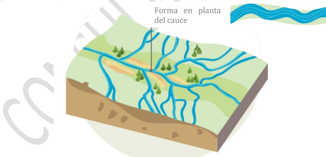
Figura 2-11. Esquemmatización de un río recto de montaña con su forma típica en planta.
